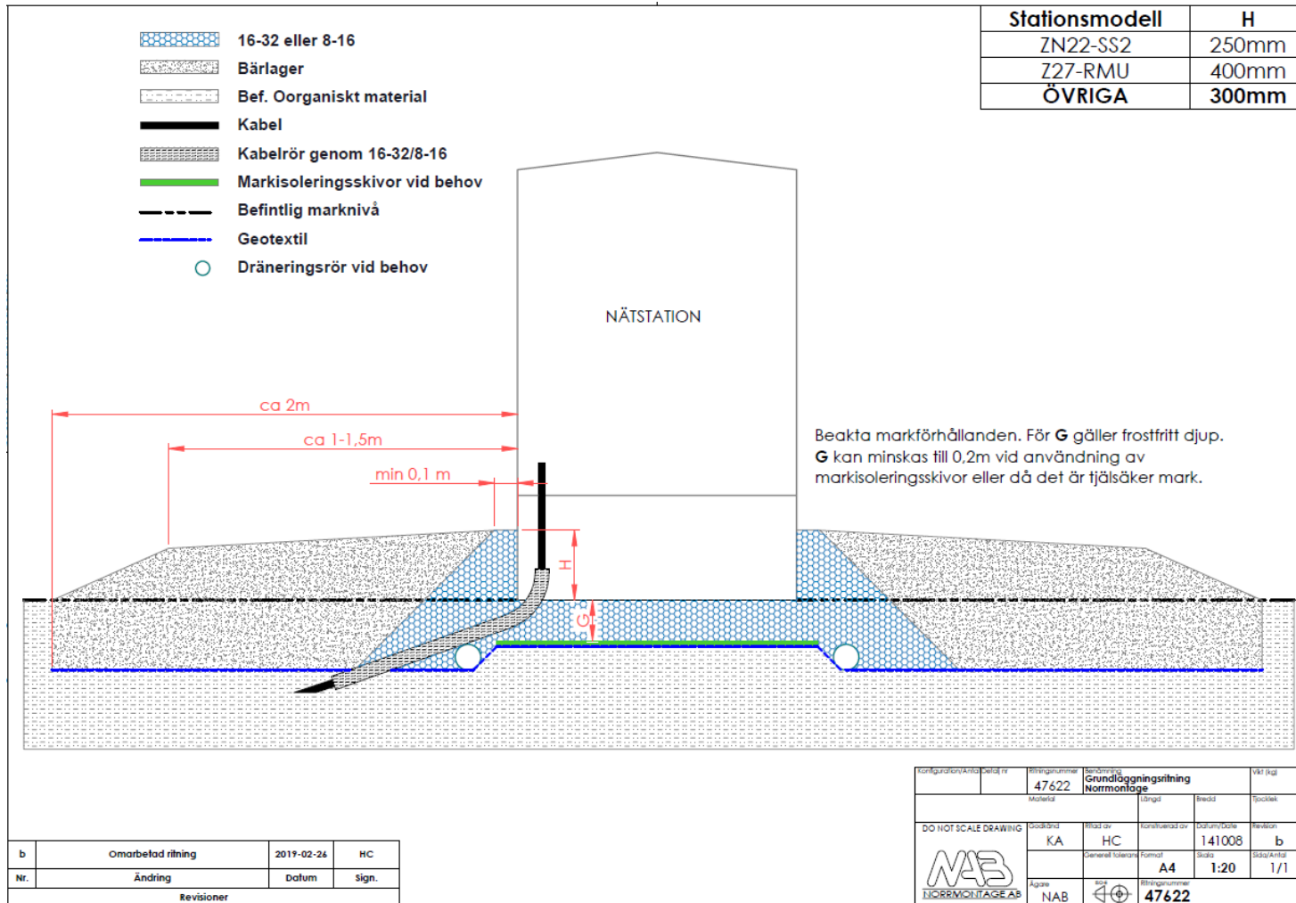
Figur 1. Grundläggning av nätstation (NAB ritning 47622b).
